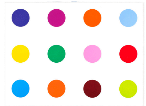
Tyloxapol
