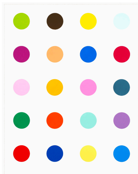
Guaiazulene
