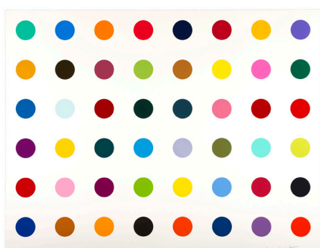
Fluoriodobenzene
